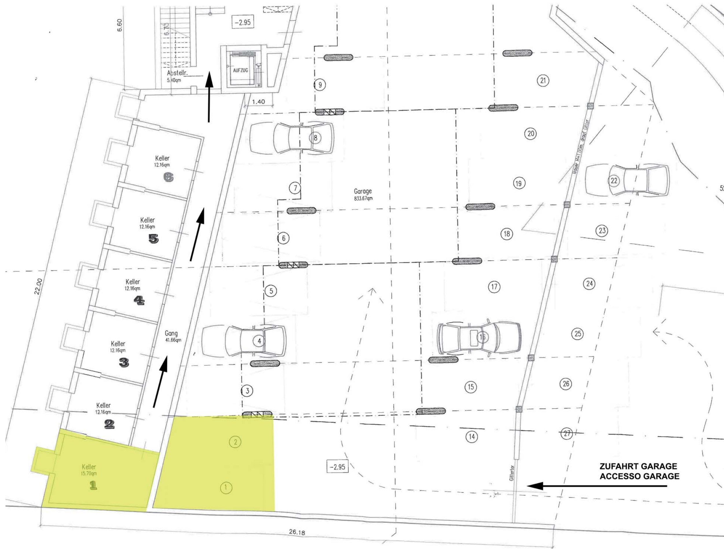
UNTERGESCHOSS - PIANO INTERRATO
